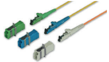
F-3000™ Simplex
