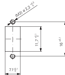
CUTOUT DIMENSIONS
